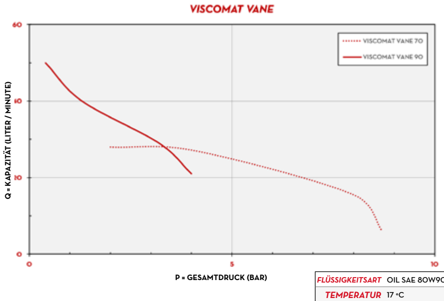
FLÜGELROTOREN
