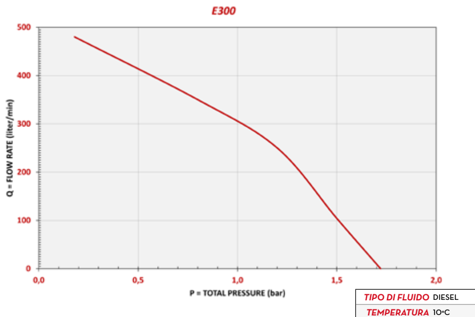
GIRANTE APERTA
