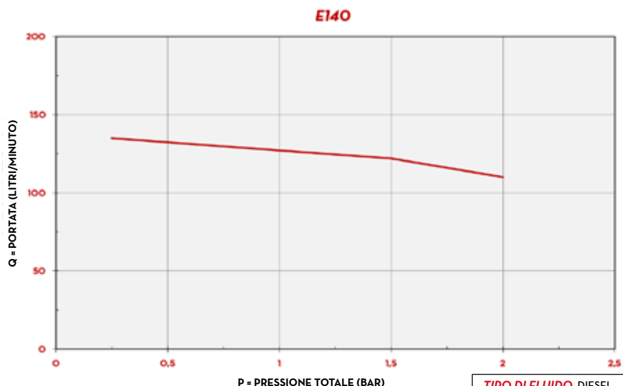
VALVOLA DI BYPASS
