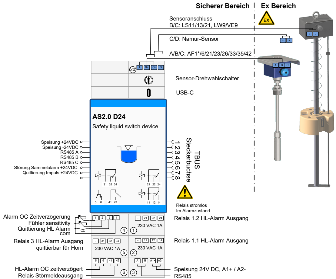
Abbildung 9 Anschlussschema AS2.0 D24 G
