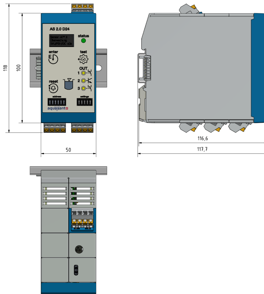
Abbildung 8 Gerätedimensionen, Auf-, Seitenansicht
