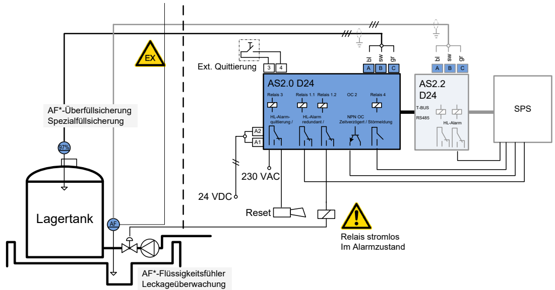
Abbildung 4 Anwendung Leckagenüberwachung Prinzipschema
