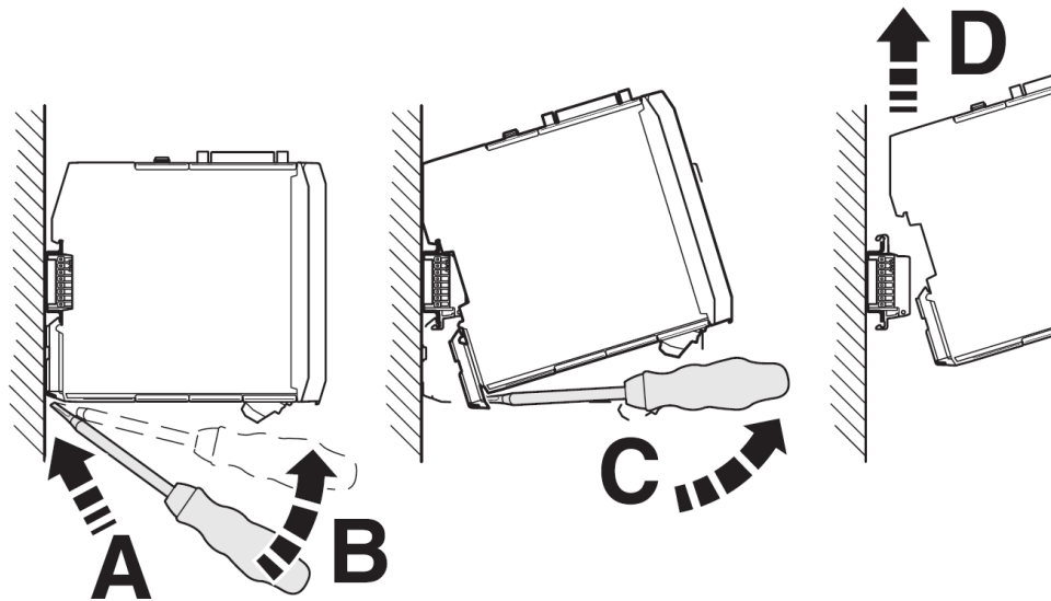
Abbildung 11 Hutschienendemontage
