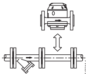
Zähler mit Flanschanschluss
