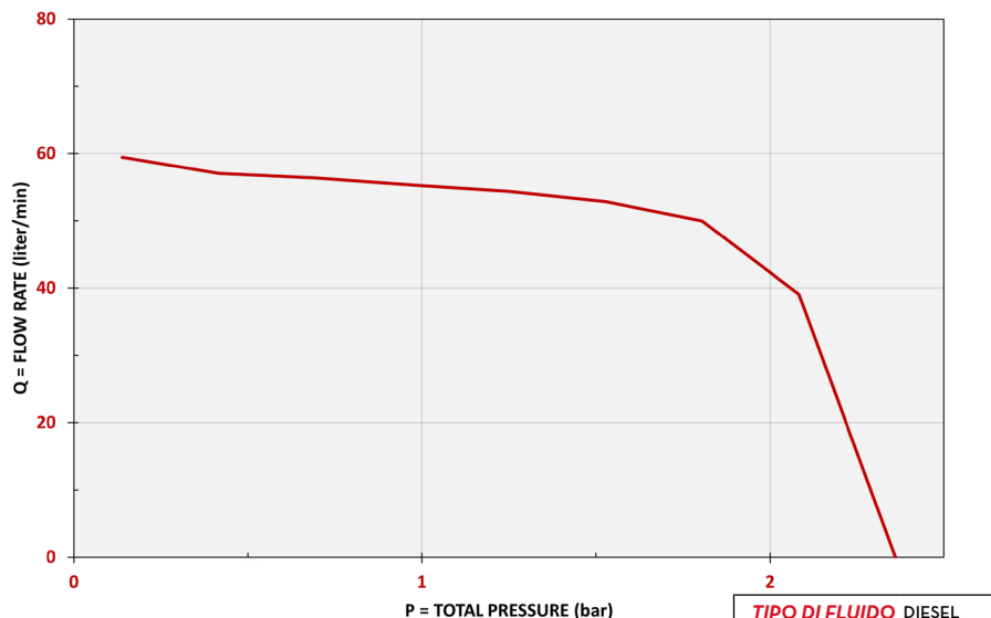
CONTALITRI DISCO NUTANTE
